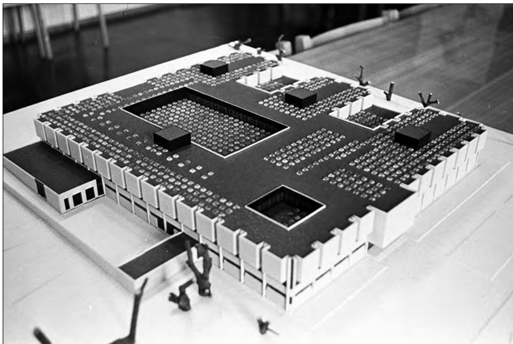
Instituudis Eesti Tööstusprojekt valminud Tartu Riikliku Ülikooli teadusliku raamatukogu uue hoone projekt. 1971. Foto: Erich Norman. EFA.204.0.87352
