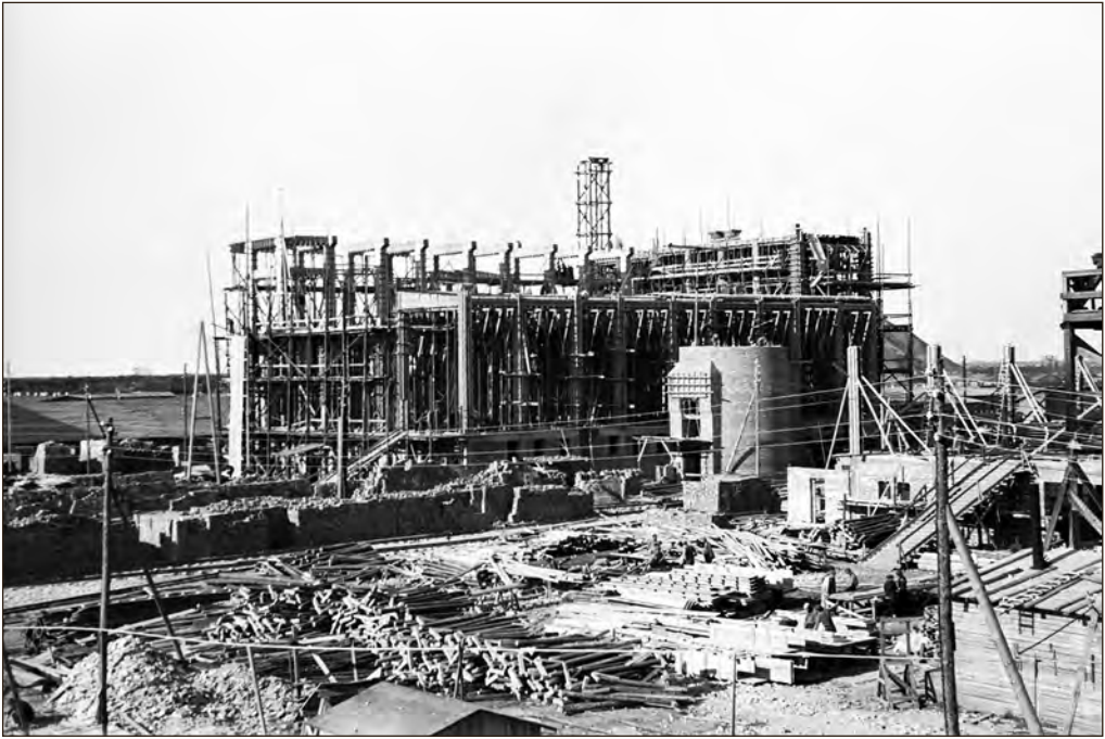
Kiviõli Põlevkivikeemia tehase ehitus 1947. aastal. Foto autor teadmata. EFA.396.0.192376
