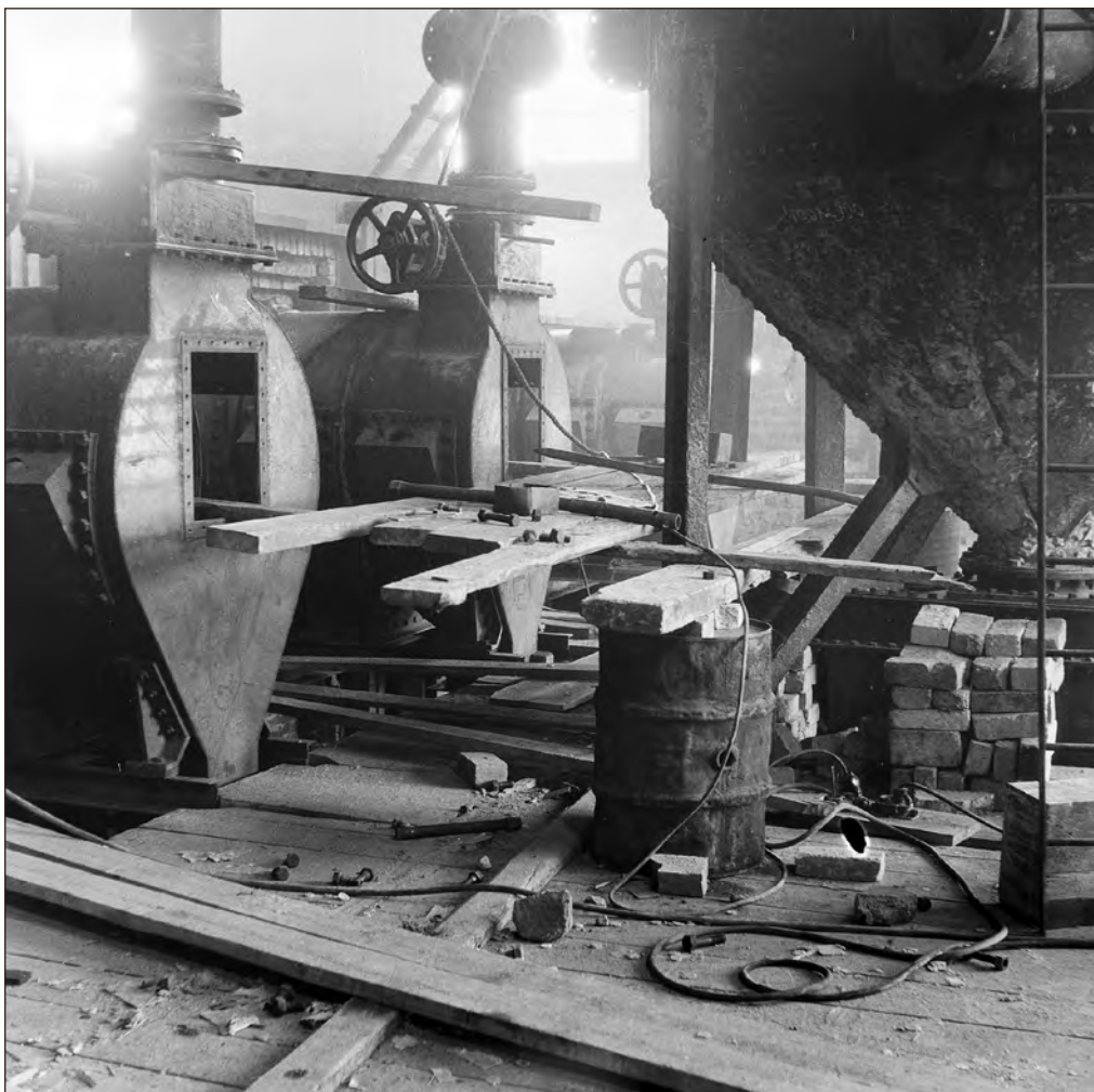
Teises maailmasõjas purustatud Kohtla Põlevkivikombinaadi Davidsoni retortide taastamine 1945. aastal. Foto autor teadmata. EFA.396.0.149485
